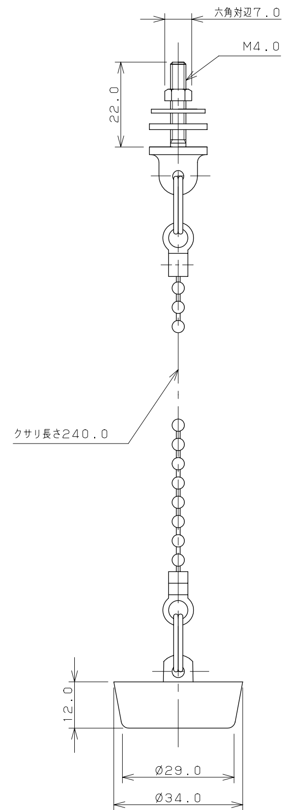
ゴム栓 (縮尺 1/1)
